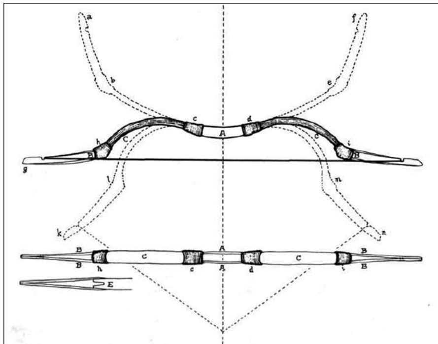
A magyar íj rekonstrukciója: a felső szaggatott vonalas rajz nyugalmi, a teltvonalas rajz ajzott, az alsó szaggatott vonalas rajz pedig feszített helyzetben mutatja be
