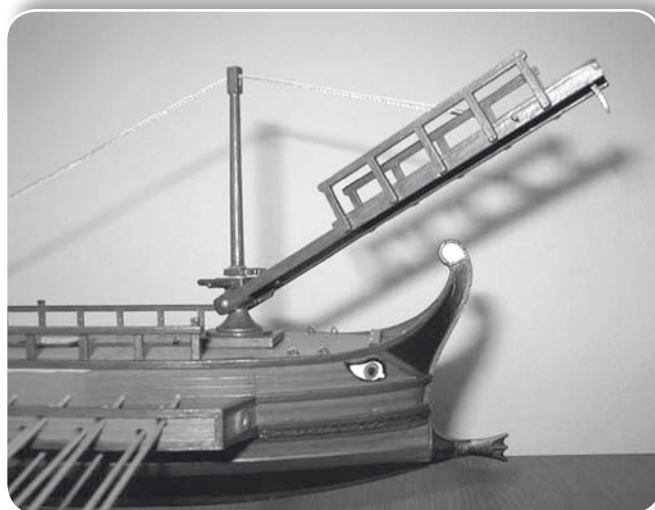
Rohamhíd
