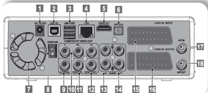
A Sencor SHR 9500 hátsó panelje
